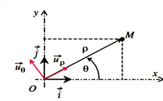
figure 2.7: Repère polaire.
