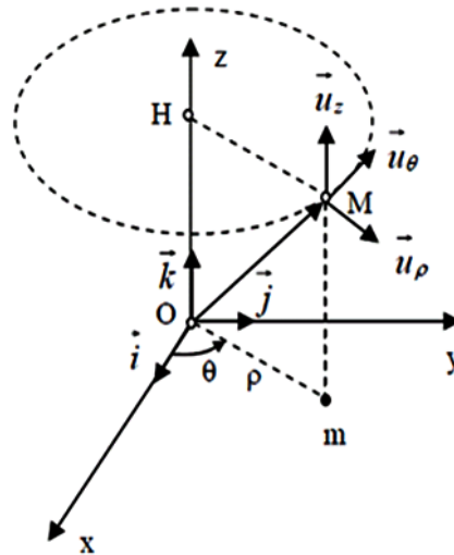
figure 2.8: Repère cylindrique.
