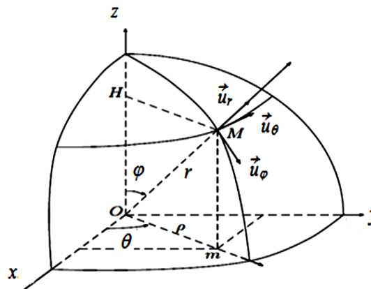
figure 2.9: Repère sphérique.
