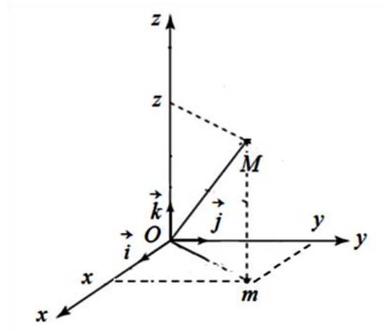
figure 2.6: Repère cartésien.
