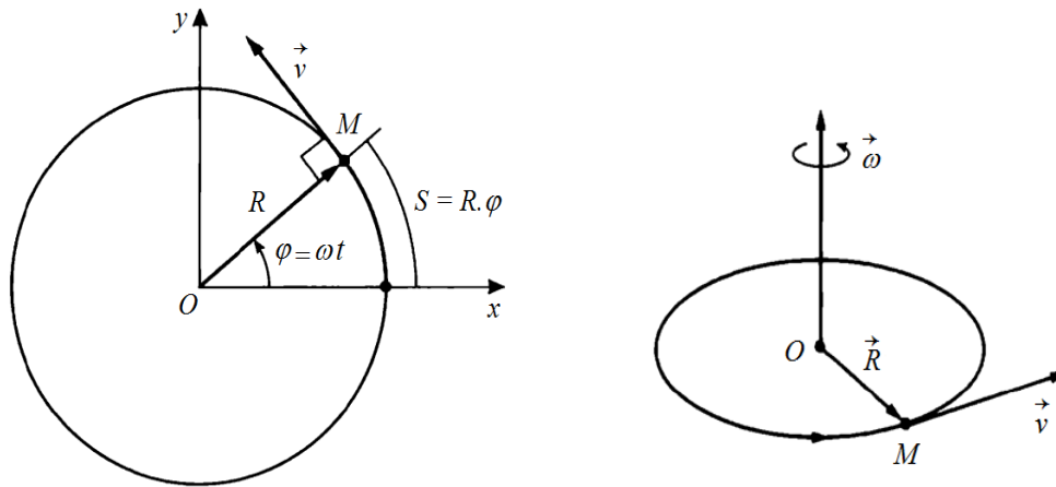
figure 3.2 : Mouvement circulaire
