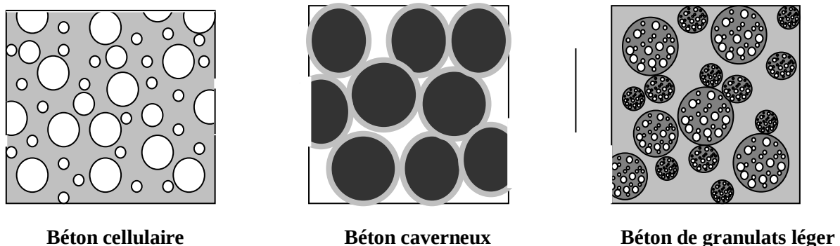
Fig . 4.2 : Les différents types de bétons légers
