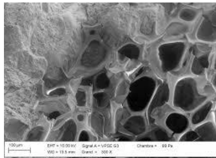
Fig ; 4.1 : MEB en béton léger
