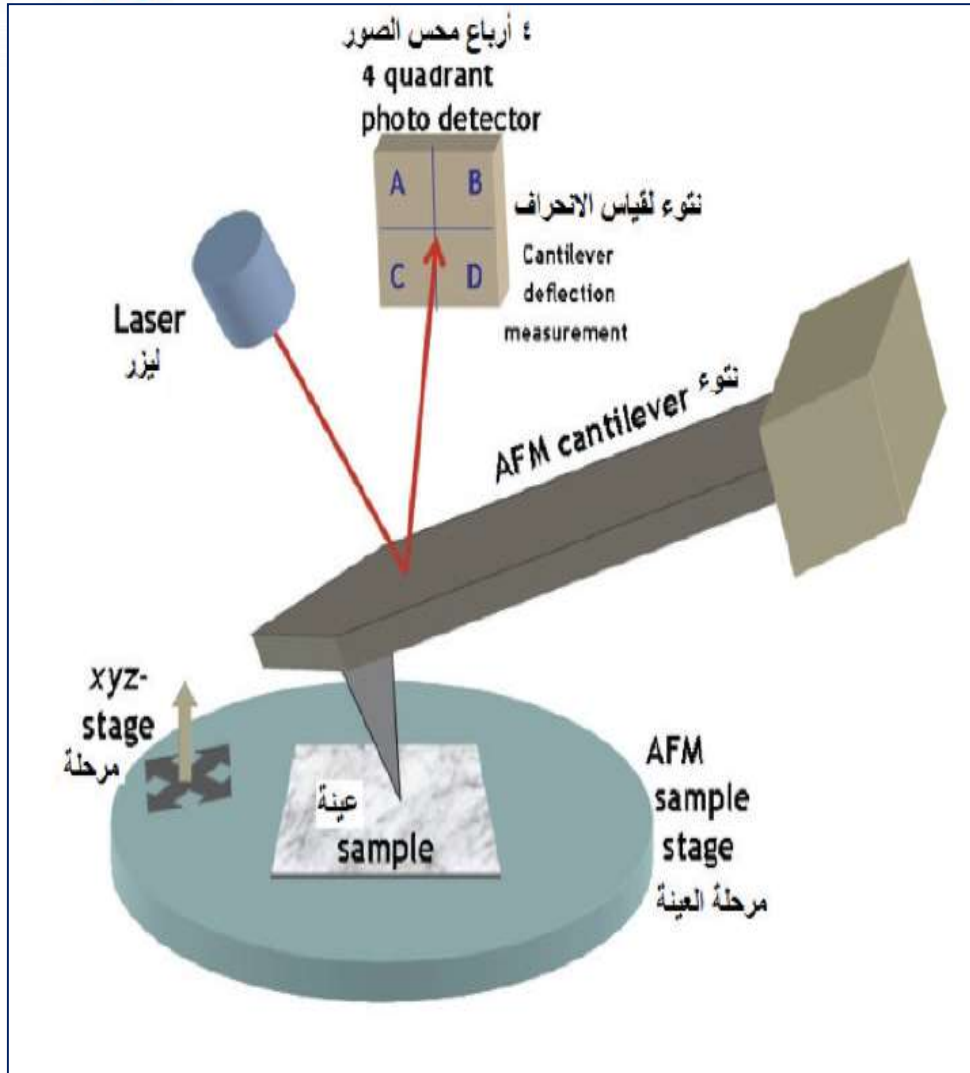
صورة توضيحية؛ لطريقة عمل مجهر القوة الذرية
