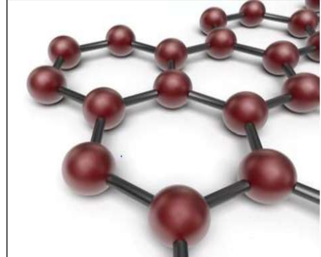
ترتيب جزيئات الكربون
