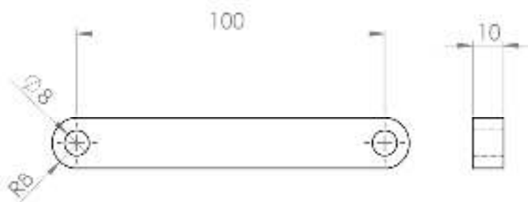
Pièce 2: Bielle
