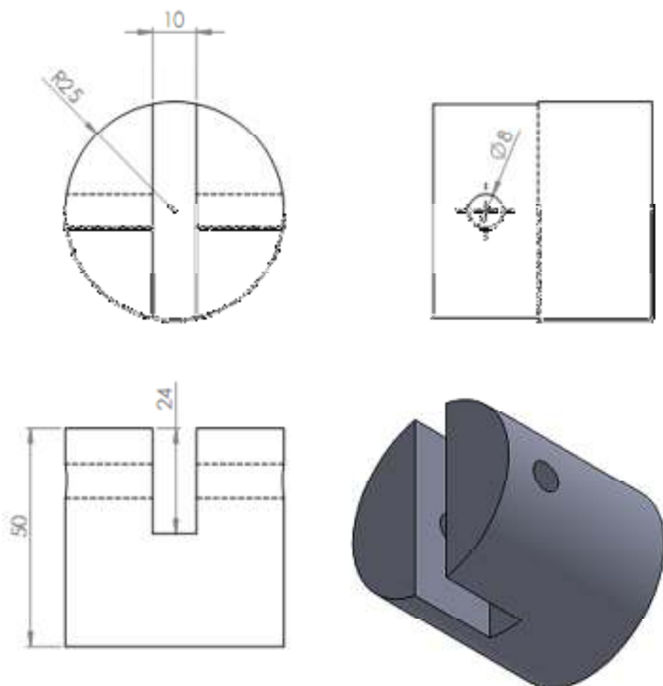
Pièce 03: Piston
