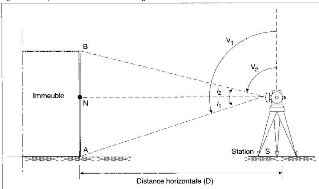
Figure 5.2 Vérification de la hauteur d'un ouvrage
