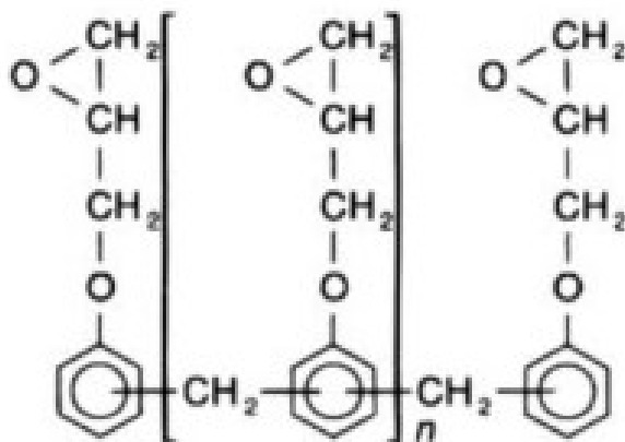
(d) Structure Époxyde phénol-novolac [Bardonnet, 1992]
