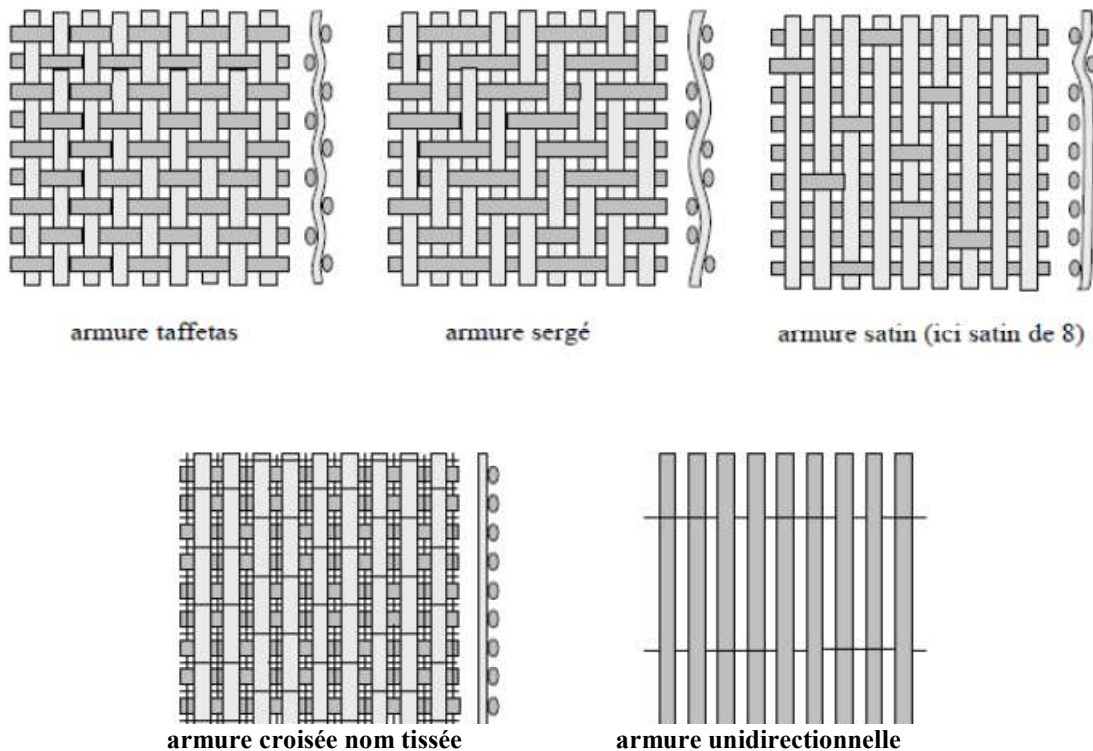
Fig.2.1 Les principaux types d'armures utilisées pour le tissage des tissus
