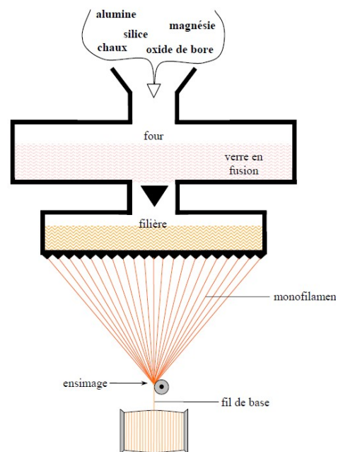
Fig 2.3 Fabrication des fibres de verre
