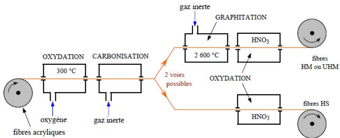
Fig.2.5 Procédés de fabrication des fibres de carbonnes
