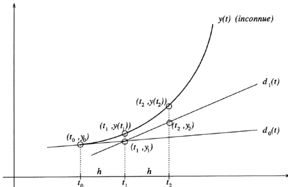
Figure 1.1. Méthode d'Euler
