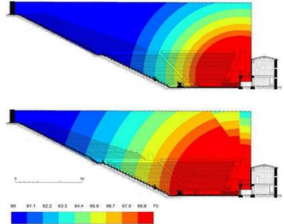
Fig. 1 3: le son direct seul (en haut), puis ajouté aux réflexions sur l'orchestra et sur la skene (en bas) ; carte du programme en transparence sur une coupe du théâtre de Priène (Source: Houtopoulos,200)
