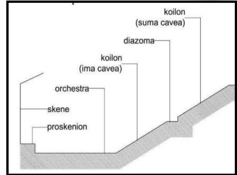
Fig 11: Coupe longitudinale du théâtre, avec une diazoma partageant les gradins ( Source: Beckers ,2007)
