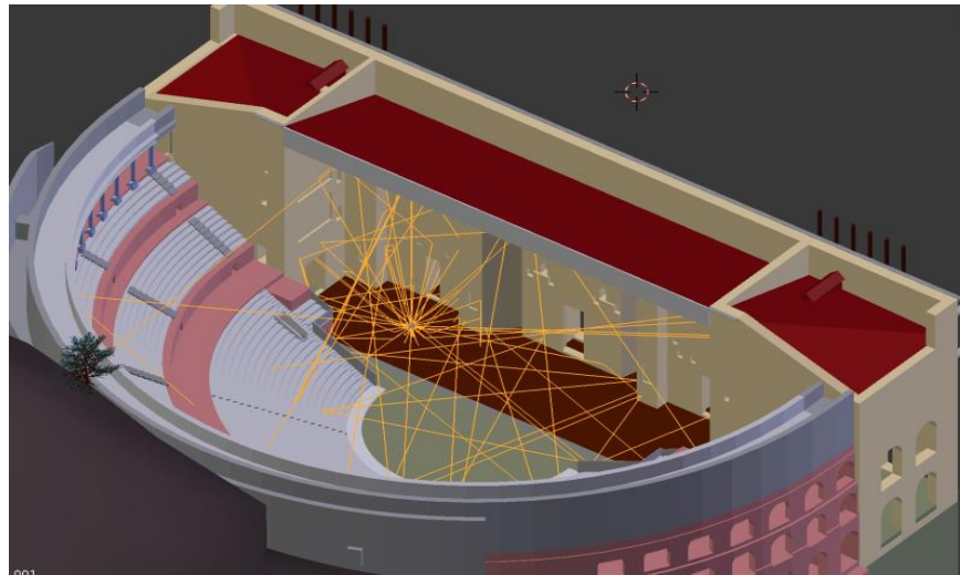
Fig 09: Visualisation d'un résultat de ray-tracing dans le théâtre antique d'Orange Source: http://www.cmap.polytechnique.fr/xaudio/acoustique.html
