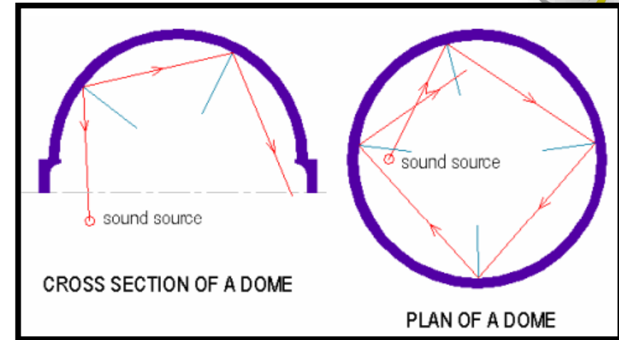
Fig 20: Comportement de l'énergie sonore dans un dôme (Source: Kayili, M. (2005))
