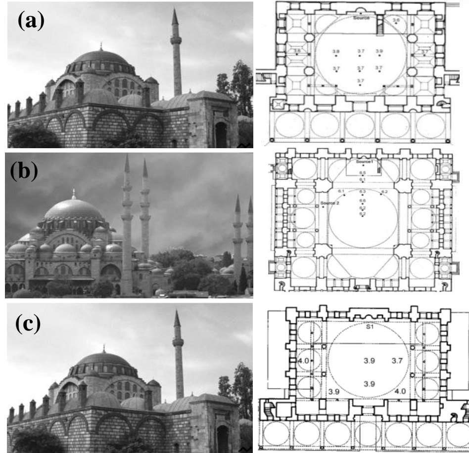
Fig 19: a) La mosquée de Rüstem Pacha (Istanbul), B) La mosquée Selimiye ou Selim (Edirne), c) Mosquée de Mihrimah Sultan (Source:Topaktas, L (2003).
