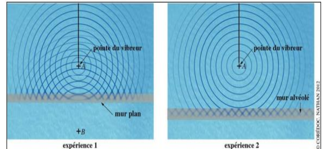
Fig 14:Modélisation de la rencontre des ondes sonores avec un mur : a) plan b) obstacle alvéolé sur le mur (Source: http://www.ac-grenoble.fr/disciplines/spc/file/ressources/Resolution_probleme/2014_TS_Spe_Son_et_musique_Acoustique_theatre_Epidaure.pdf )
