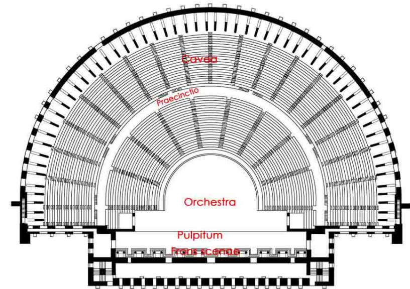
Fig 07:Plan du théâtre romain à Aspendos Aspendos, Belkiz ou moderne, la Turquie. Après Wilhelm Dörpfeld (Source: https://www.alamyimages.fr/photo-image-plan-du-theatre-romain-a-aspendos-aspendos-belkiz-ou-moderne-la-turquie-apres-wilhelm-dorpfeld-75339986.html )
