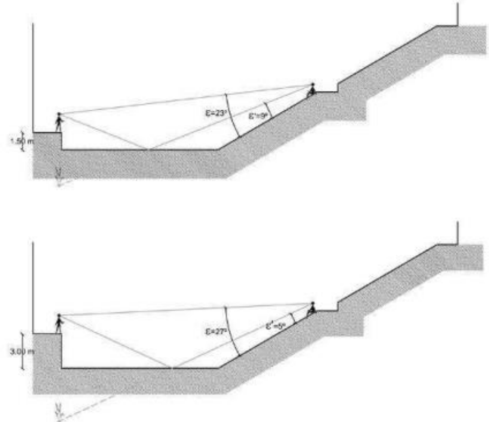
Fig. 12 : Si l'on hausse le proskenion, l'angle \epsilon d'incidence du son direct au spectateur croît, mais l'angle \epsilon' d'incidence du son réfléchi décroît. (( Source: Beckers ,2007)
