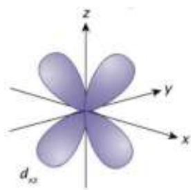
\Psi_{3,2,2}
