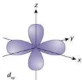
\Psi_{3,2,1}
