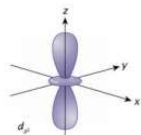
\Psi_{3,2,0}
