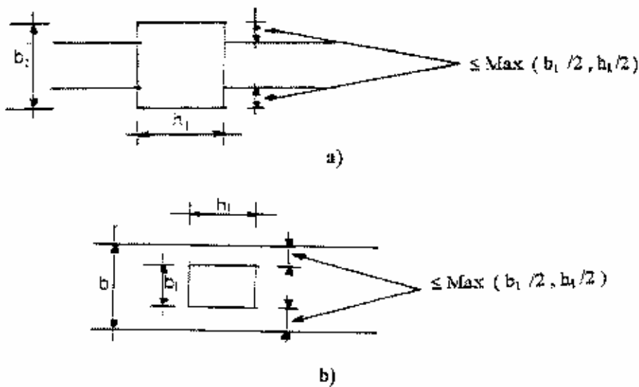
Fig 7.4 : Dimensions à respecter par les poutres
