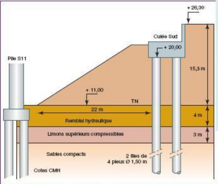
Fig. 4 - Coupe transversale schématique au droit de la culée Sud.
