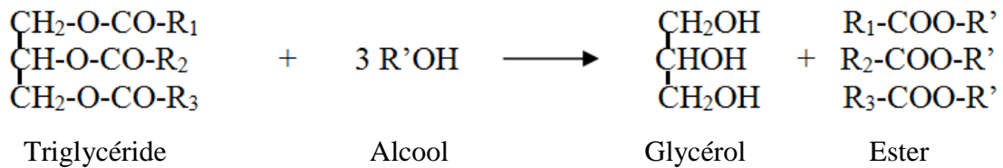
Figure 39 : alcoololyse d'un triglycéride.
