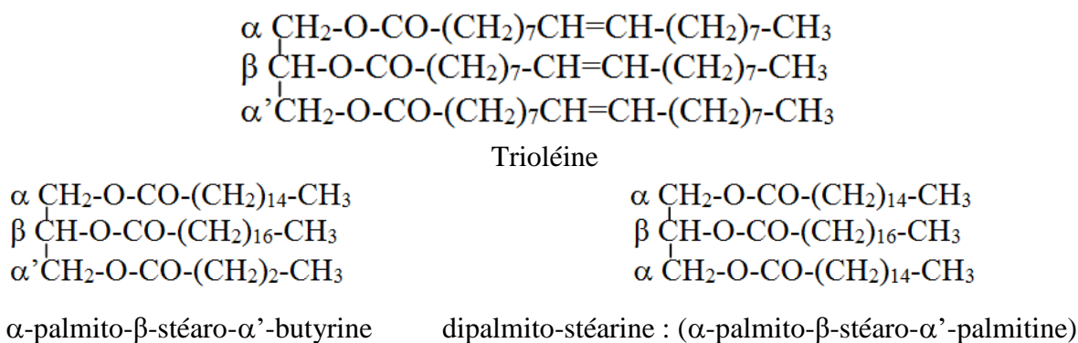
Figure 35 : exemples de triglycéride.
