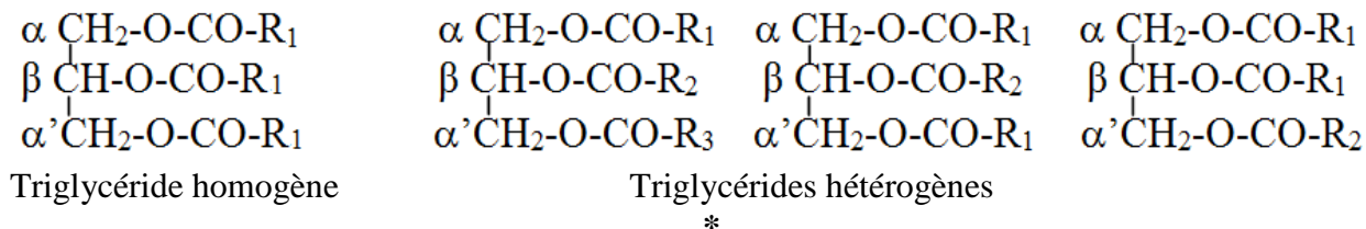
Figure 33 : structure d'un triglycéride.
