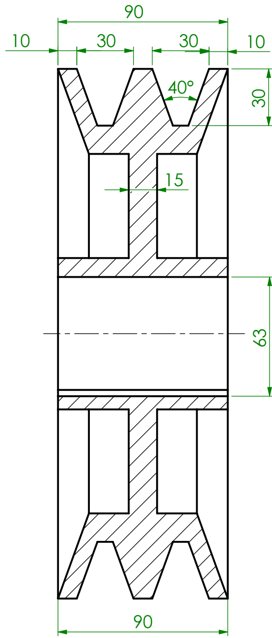
COUPE A-A
